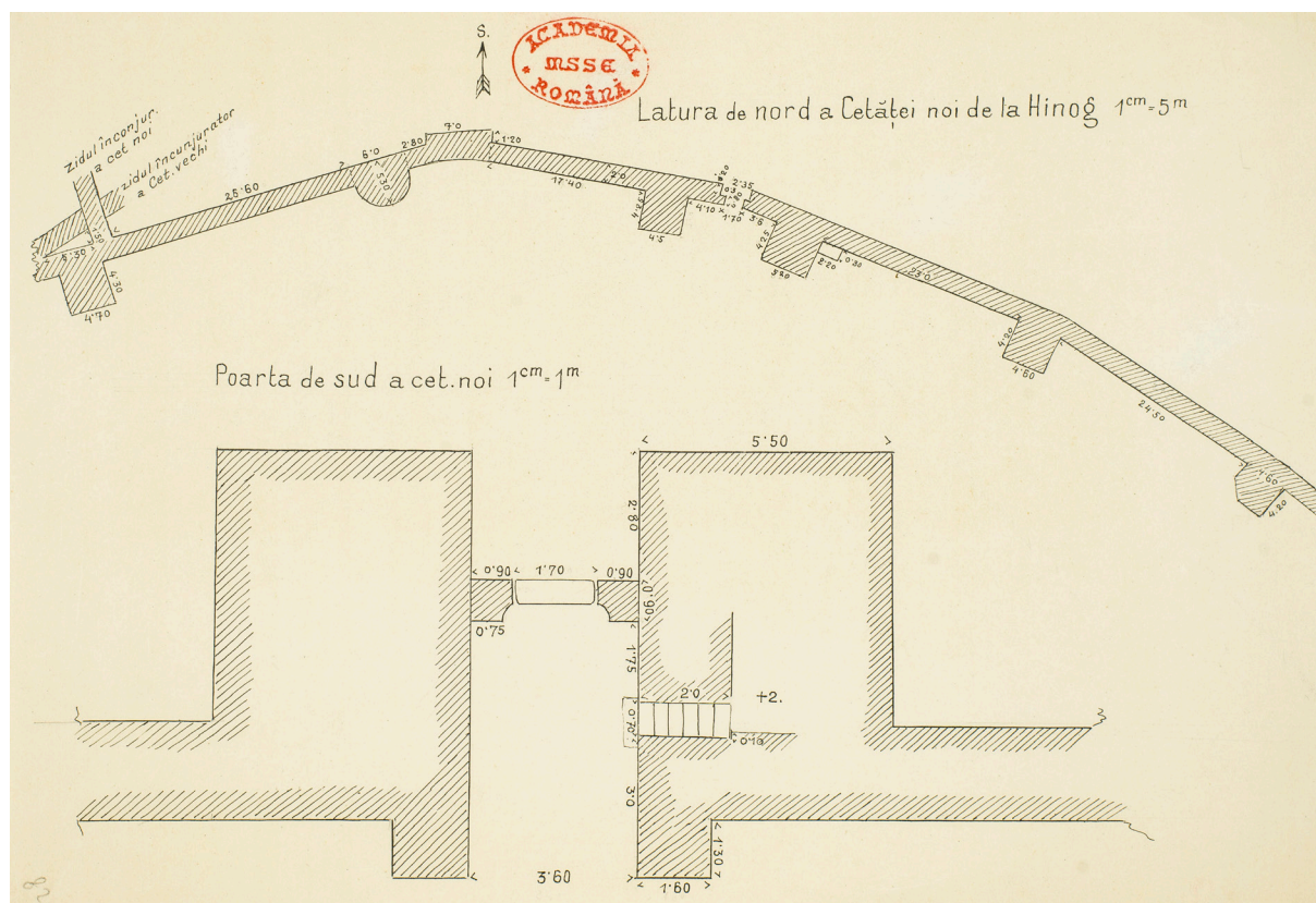
Fig. 26. Latura de N a cetății noi; poarta principală (de S) a cetății noi. BAR, Mapa Pamfil Polonic Varia I , desen 82.
