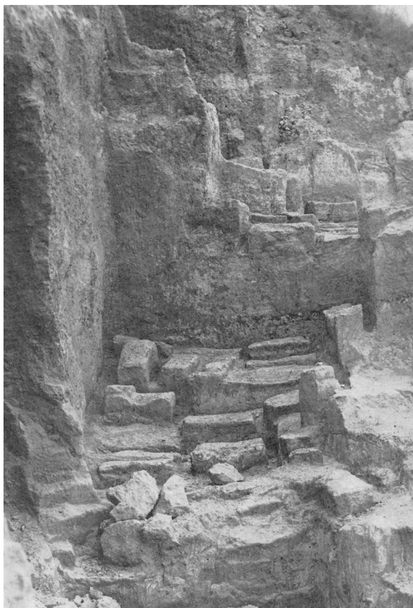
Fig. 32. Cariera de piatră de la Axiopolis (excavațiunea 4). Miclea, Florescu 1980, fig. 417.
