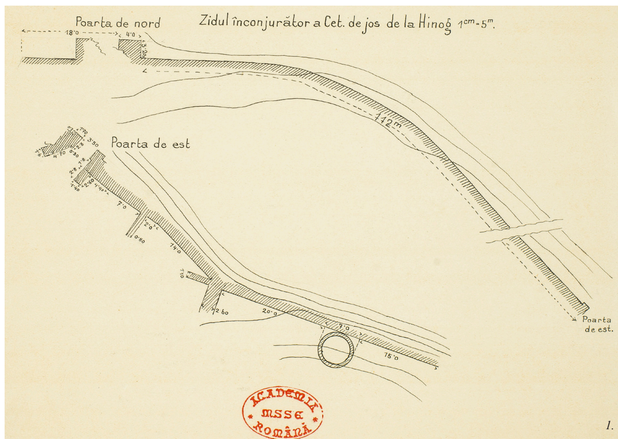
Fig. 21. 1. Incinta de N și E a cetății B (de jos) cu detalii asupra porților. BAR, Mapa Pamfil Polonic Varia I, desen 80. 2. Poarta de E a cetății B (de jos). BAR, Mapa Pamfil Polonic Varia I, desen 87.
