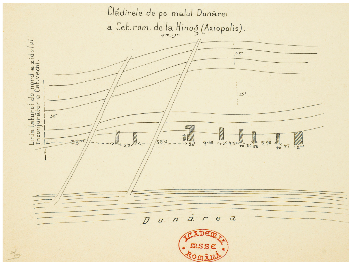
Fig. 20. Ziduri de clădiri (instalația portuară ?) perpendiculare față de malul Dunării, la baza Dealului Hinoș (cetatea A). BAR, Mapa Pamfil Polonic Varia I, desen 79.
