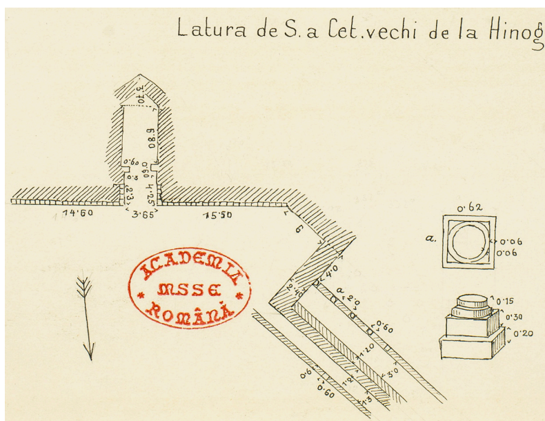
Fig. 12. Latura de S a cetății vechi (A) de la Hinog. BAR, Mapa Pamfil Polonic Varia I, desen 80. BAR, Mapa Pamfil Polonic Varia I, desen 77 (jos).
