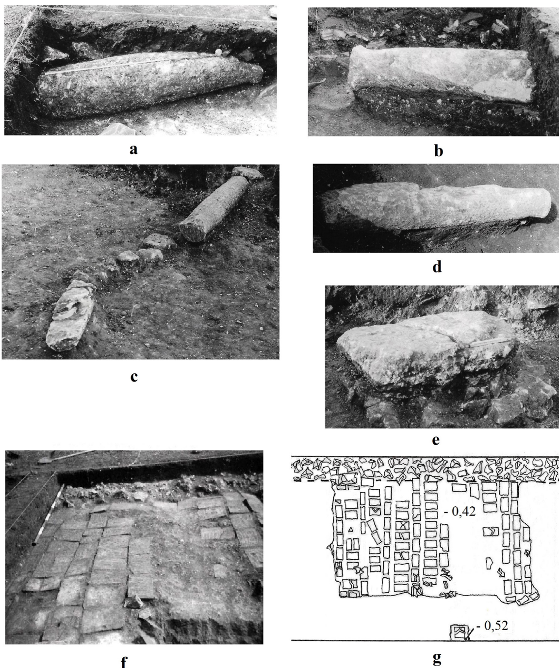
Figure 4. Coloane din cohors quingenaria (retentura sinistra) (a-e) și aranjamentul cu cărămizi din spațiul Sp. 1 (f-g).
