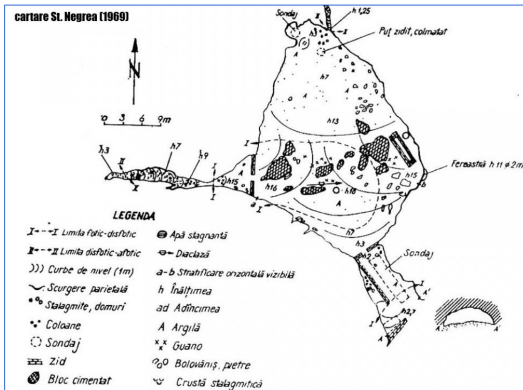
Fig. 2 – Planul Peșterii Veterani realizat la finalul investigațiilor „Grupului de cercetări Porțile de Fier”, https://speologie.org/pestera-veterani * Plan of the Veterani Cave made at the end of the investigations of the „Iron Gates Research Group”, https://speologie.org/pestera-veterani .
